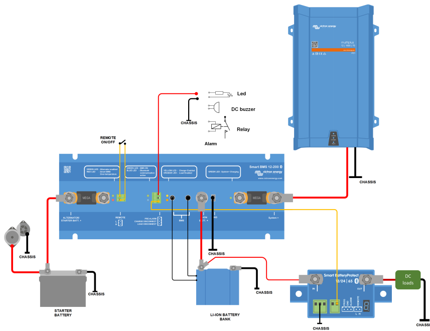
Afbeelding 2: Toepassingsvoorbeeld met een MultiPlus en een BatteryProtect
