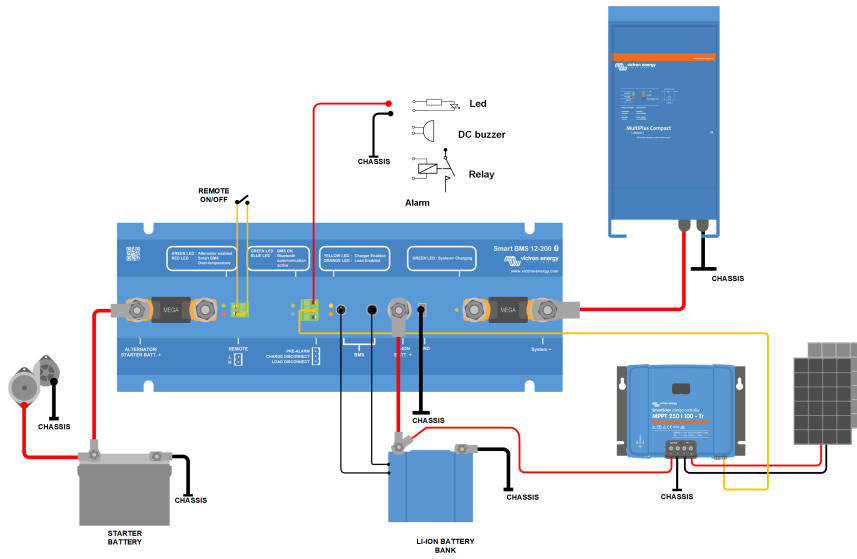
Afbeelding 1: Toepassingsvoorbeeld met een MultiPlus en een MPPT
