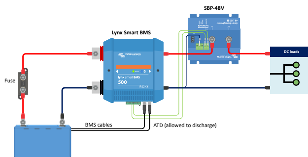
Smart BatteryProtect in Li-ion modus geregeld door ATD vanuit een Lynx Smart BMS
