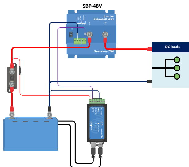
Smart BatteryProtect gebruikt de elektrisch vermogen-ontkoppeling van een smallBMS
