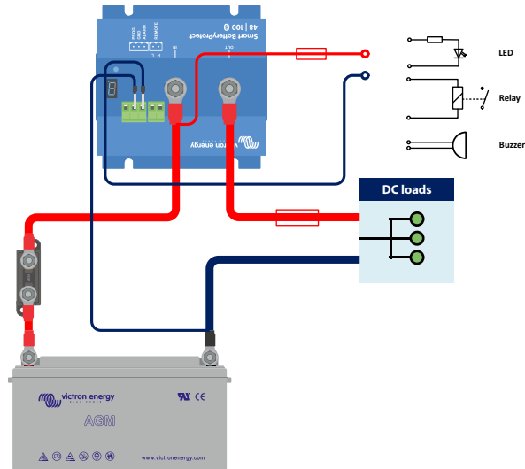
Bedraden van een led, zoemer, of relais aan de Smart BatteryProtect uitvoer
