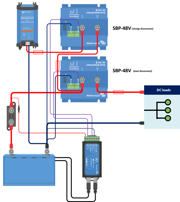
Twee Smart BatteryProtects nemen het beheer over van een lader en elektrisch vermogen-circuit
