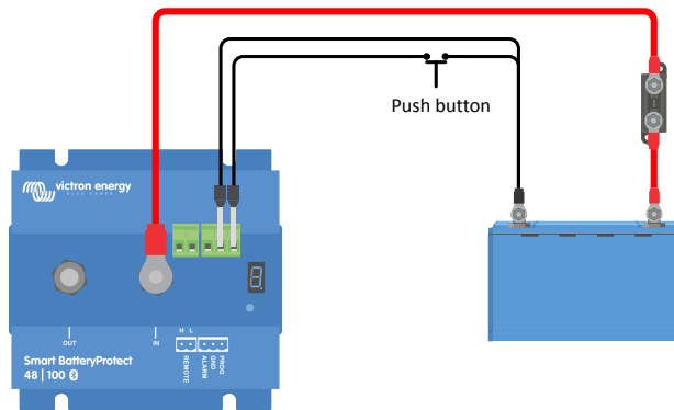
Druktoets bedraad om het Smart BatteryProtect te programmeren
