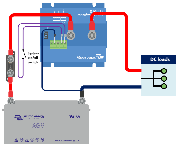
Smart BatteryProtect met remote aan/uit-schakelaar
