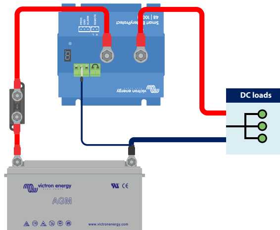
Smart BatteryProtect in een eenvoudig systeem met kabellus tussen L en H-invoer (fabrieksstandaard)
