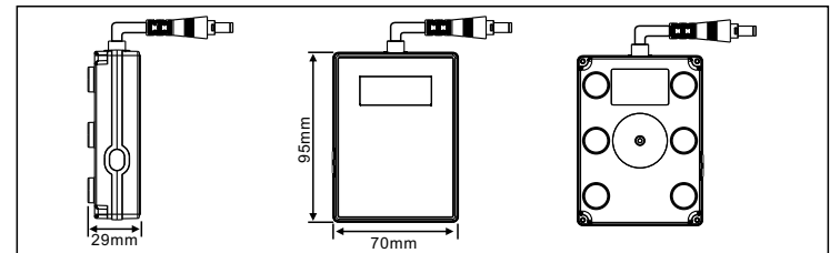
Shell dimension(mm)
