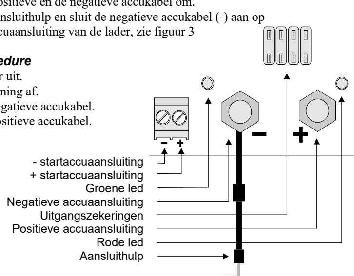
Figuur 3. Positie van de accu- aansluitingen.
