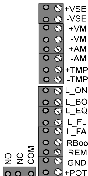
Figuur 8. Positie van de externe aansluitingen.
