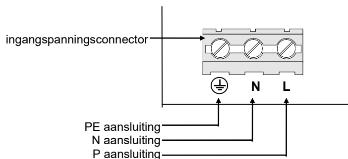
Figuur 4. Positie van de netspanningsconnector.
