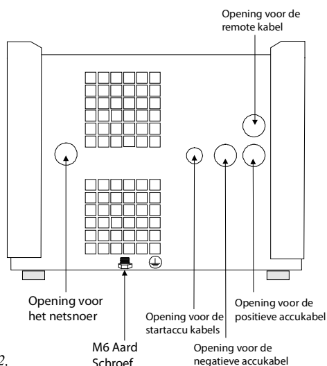
Figuur 2, Positie van de aansluit openingen
