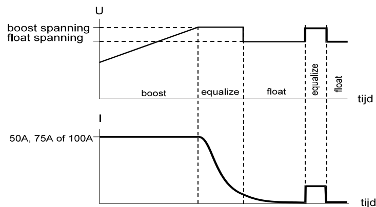
Figuur 1. De IUoUo laadkarakteristiek.
