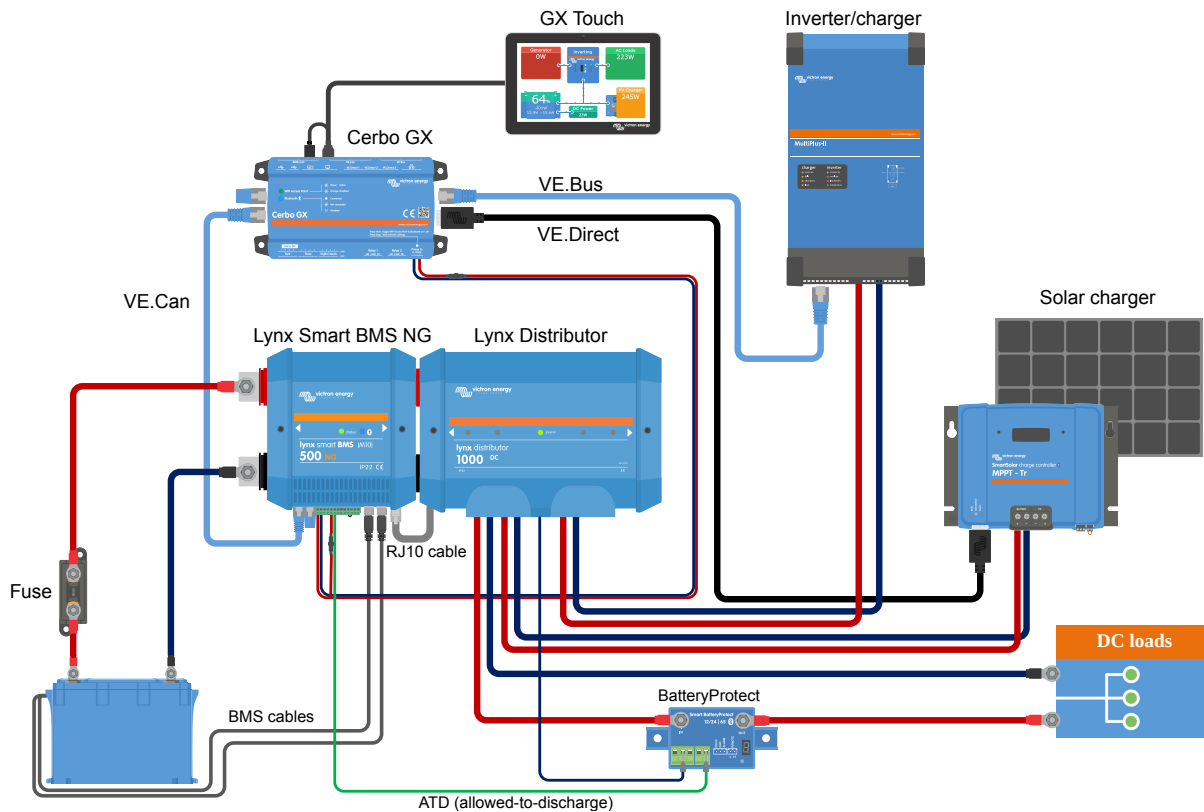
Systeem met een Lynx Smart BMS NG en een enkele Lynx Distributor
