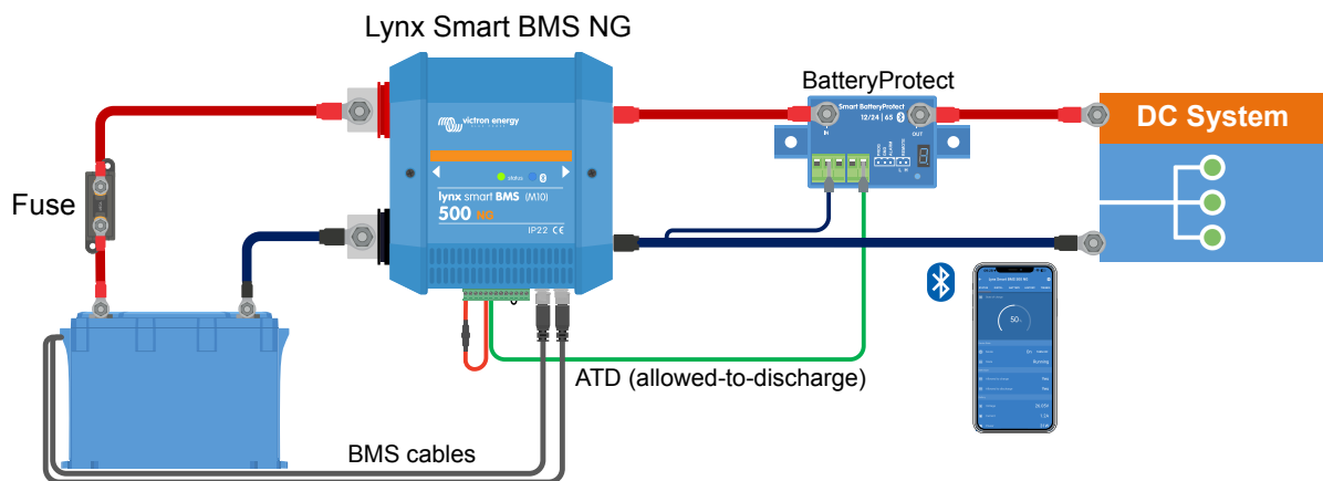
Systeem met een Lynx Smart BMS NG, zonder andere Lynx modules en GX apparaat.
