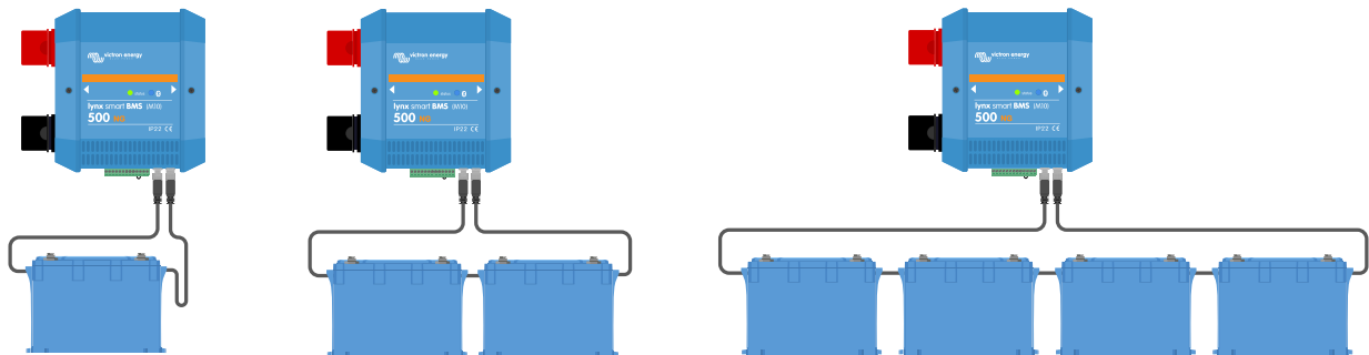
Voorbeelden van BMS kabelverbindingen Lynx Smart BMS NG accu
