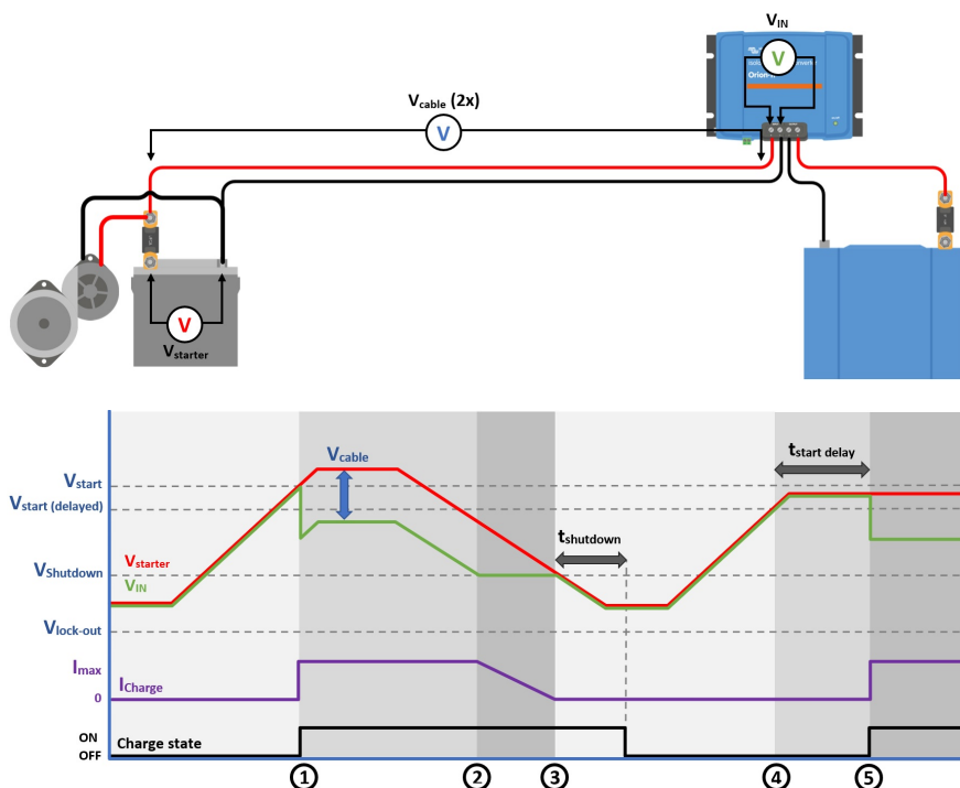
Afbeelding 8: Werking motoruitschakelingsdetectie
