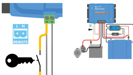
Afbeelding 4: Overschrijven detectie motoruitschakeling aansluitingsdiagram
