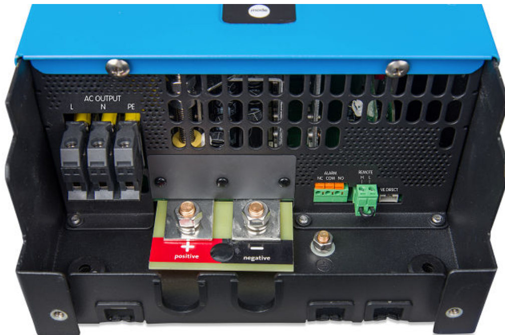
Aansluitingen 1600 VA-model
