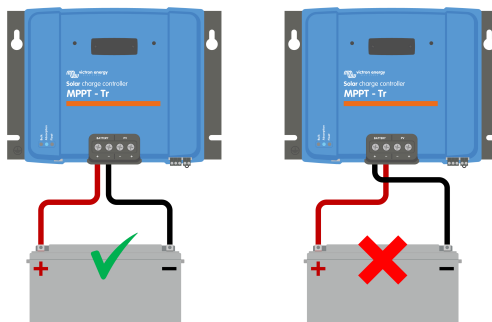
Voorbeelden van juiste en onjuiste (omgekeerde) accupolariteit.
